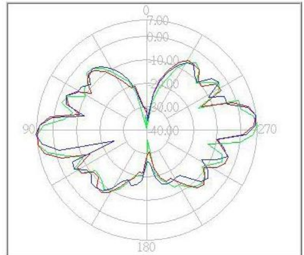
E-Plane
