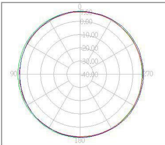
H-Plane
