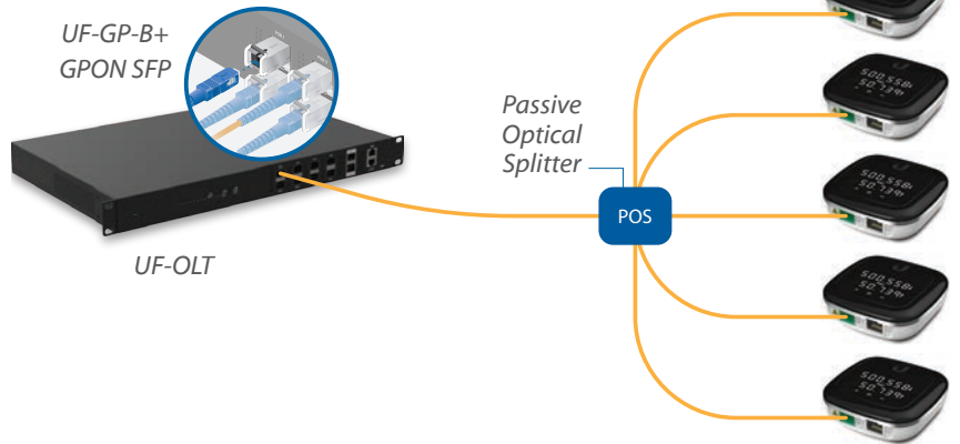
Up to 128 UF-Nano per OLT GPON Port
